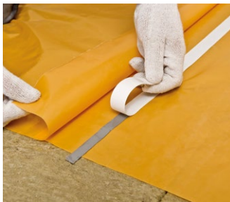
Рис. 3. Монтаж и проклейка нахлестов пароизоляционной пленки
